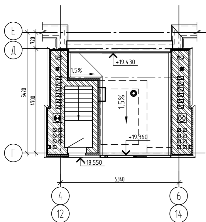
Фрагмент плана выхода на кровлю.
