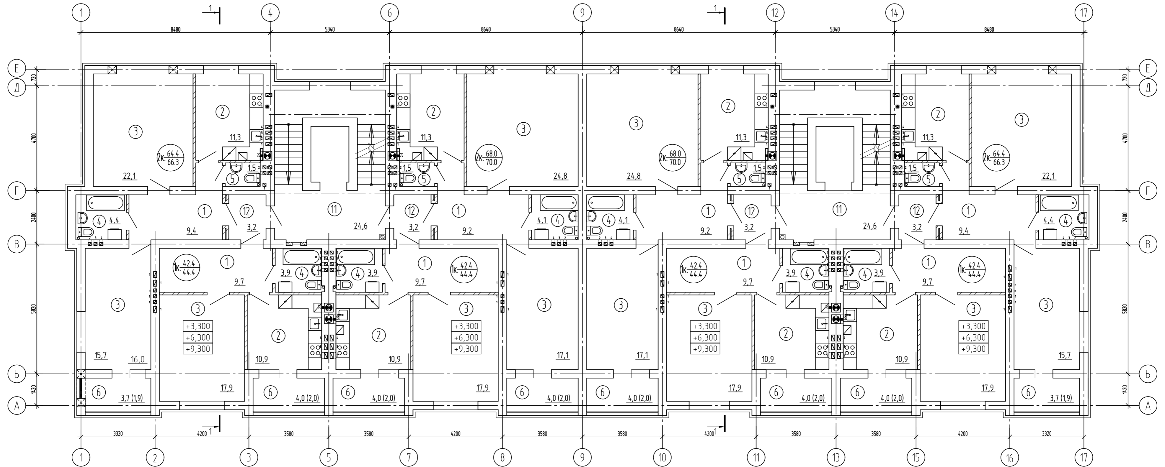
Экспликация помещений 2-4 этажа
